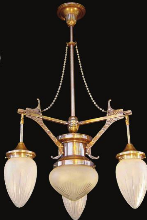
3 armed chandelier VIII. ↑80 cm ↔52 cm 4 x 75 W E27 3,8 Kg
