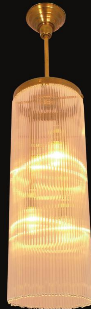
Pendant V. ↕ 80 cm ↔ 20 cm 4 x 60 W E14 1 Kg
